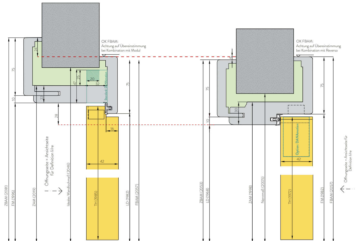
Abbildung: Gegenüberstellung Lotschnitt Systematik MODUL REVERSO vs. MODUL.
