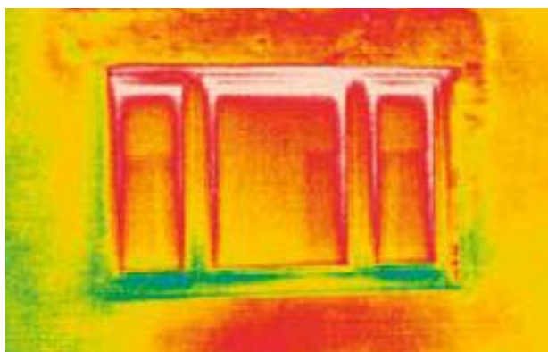
Vor der Renovierung (Rot zeigt den Wärmeverlust)
