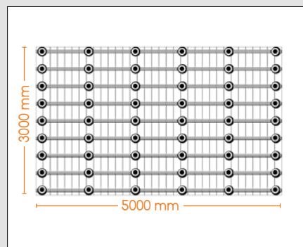
BIG-Isostep (Alu) 54 Terrassenlager Abstand Auflage- punkte max. 110 cm
