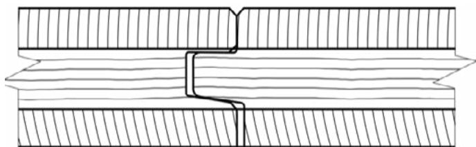
Keil-Nut-Feder mit Fase
