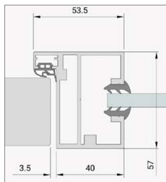
Zwischen-Wand-Montage stumpfe Holztür mit Seitenteil/Oberlicht
