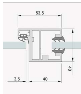
Zwischen-Wand-Montage mit festem Seitenteil
