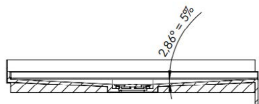
SCHNITT A-A
