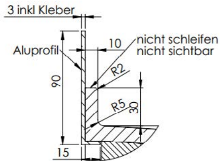
DETAIL C MAßSTAB 1 : 2
